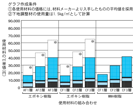
■図1 連続繊維補強工法に用いる材料の㎡単価
